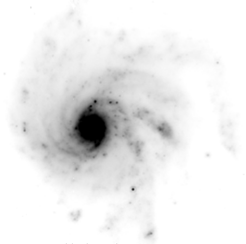
H-band
